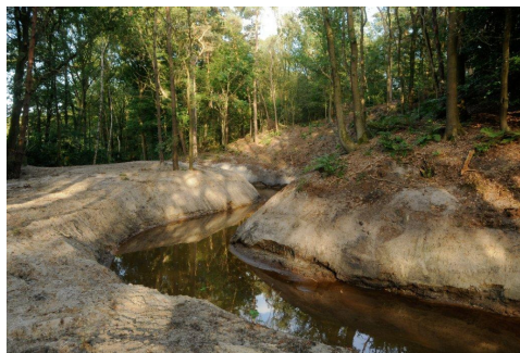
Lingsforterbeek nach Renaturierungsmaßnahmen
